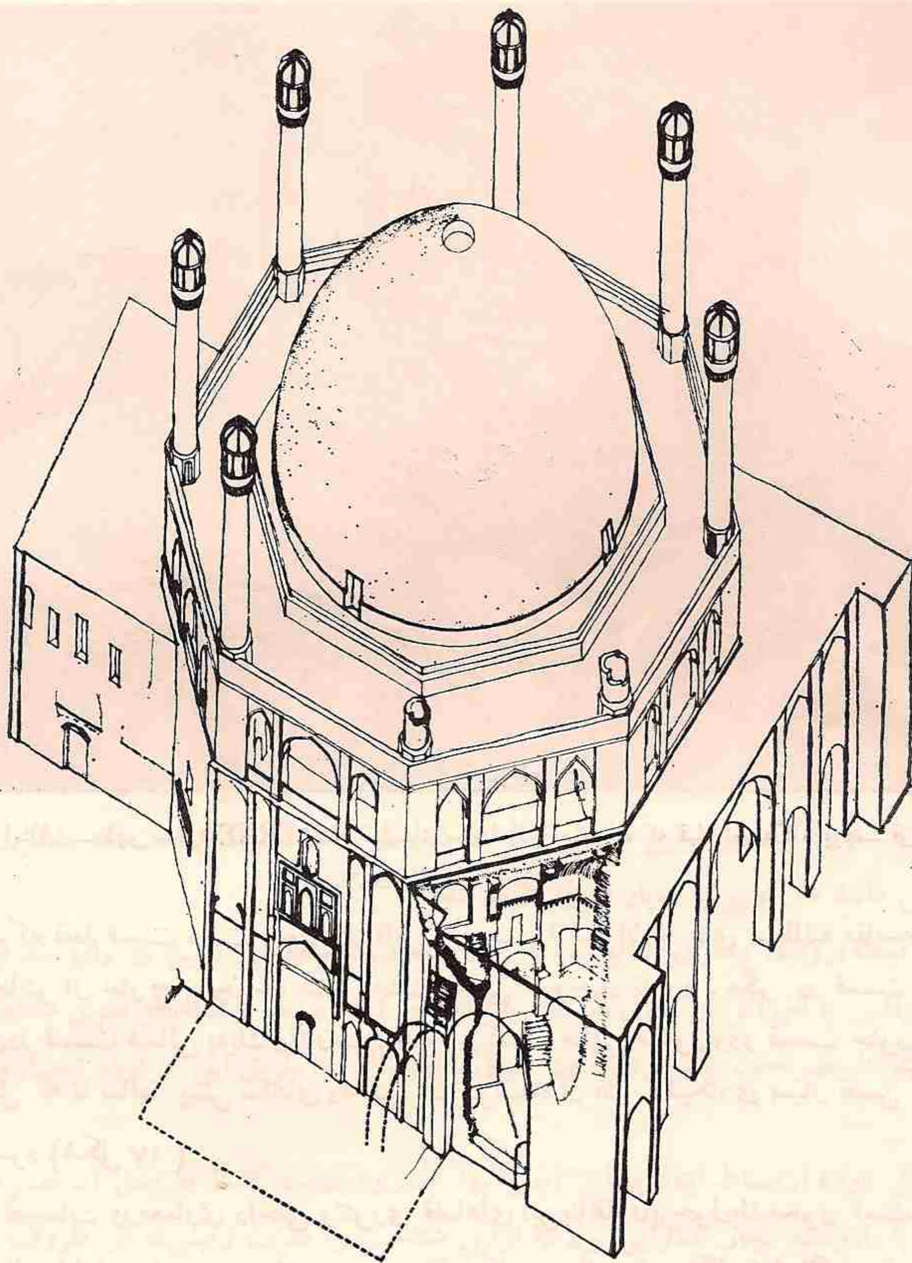
۲۱ - سلطانیه - مقبره الجایتو - بازسازی پیشنهادی دالان جلوخان بنا
