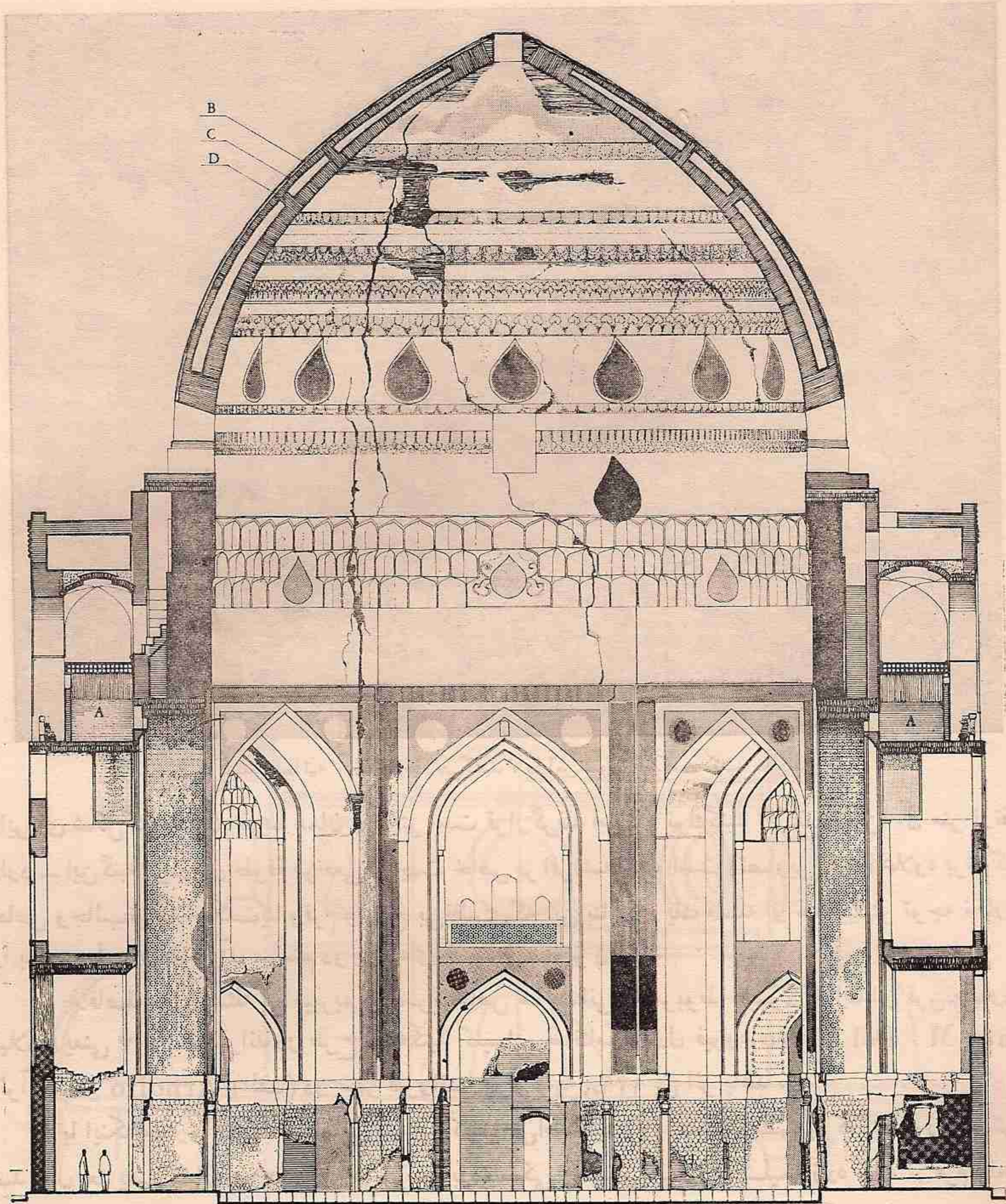
۵ - گنبد سلطانه ، مقطع عرضی
