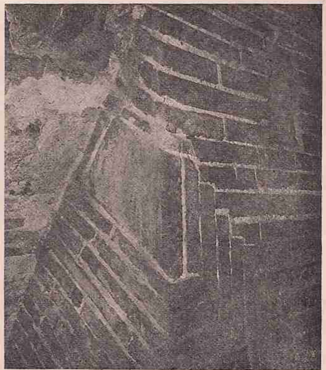
۳۸ فلورانس - گنبد سانتاماریادلفیوره - نحوه کاربرد آجر
